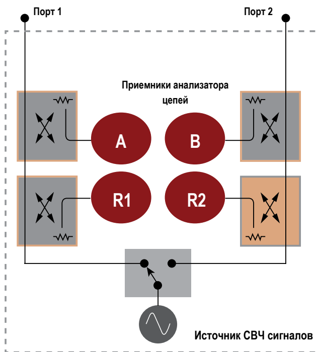
Архитектура векторных СВЧ-анализаторов цепей FieldFox
