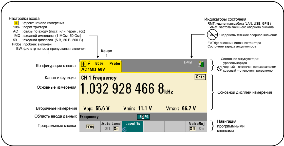
Рисунок 1-2 Дисплей 53210A
